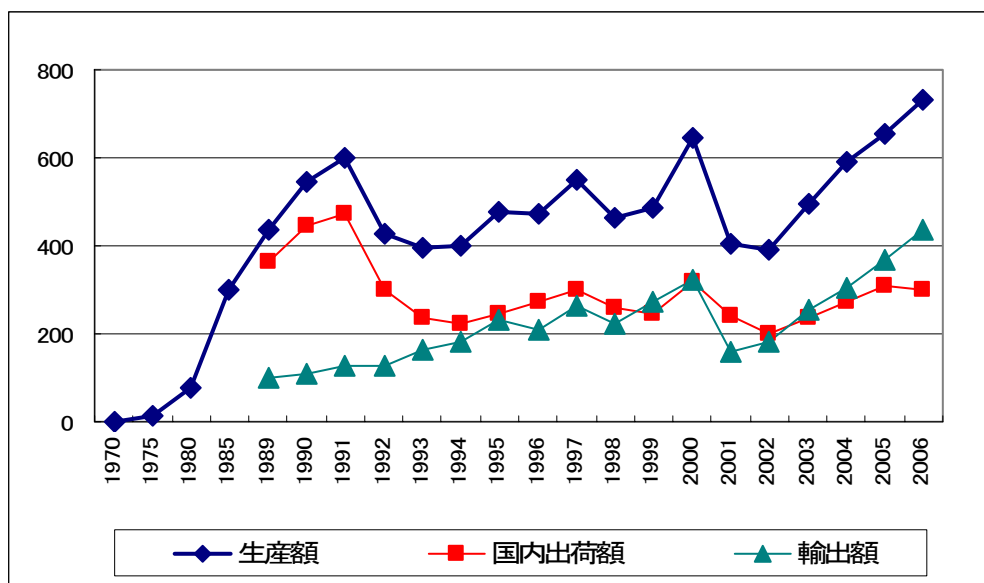
図 1. 日本における産業用ロボットの生産額，国内出荷額，輸出額（単位：10 億円）
