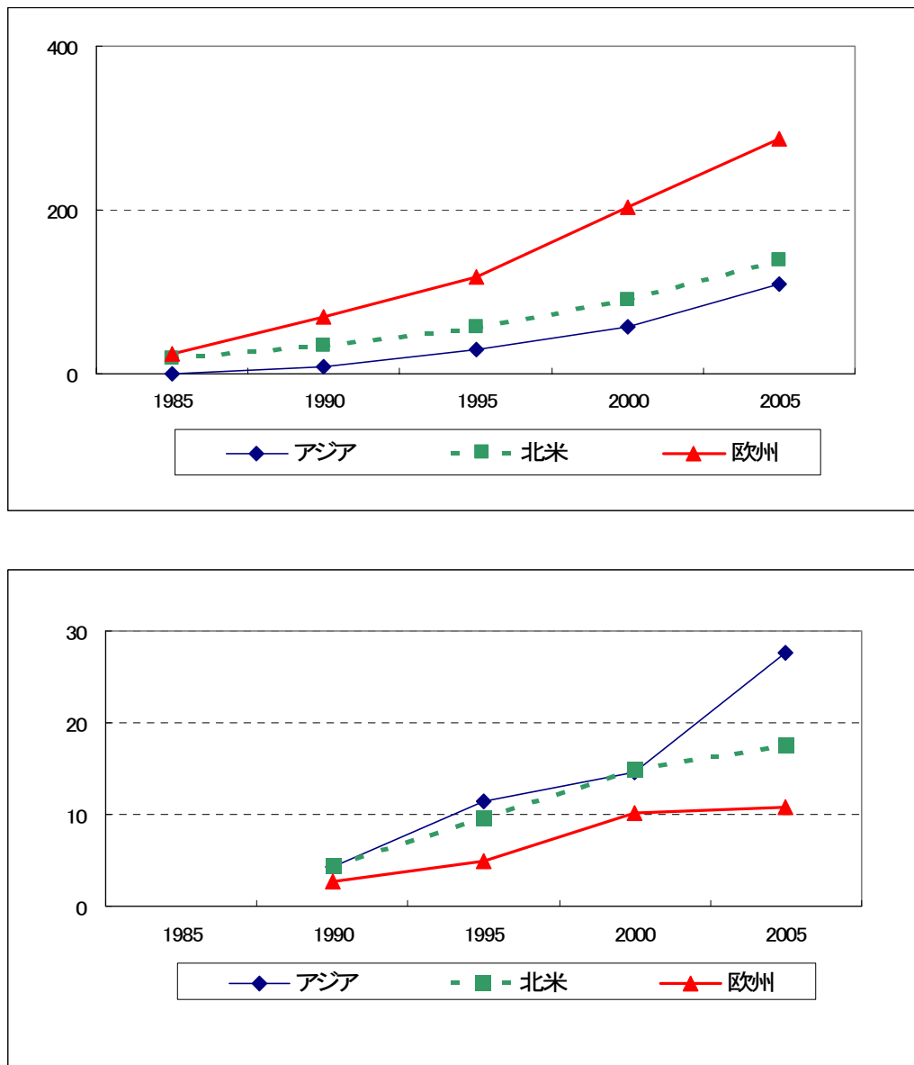
図 6. 地域別ロボット稼働台数と日本からの輸出台数（単位：1,000 台）
